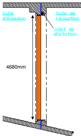
Coupe Horizontale
